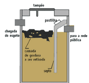
Caixa de Gordura esquema de funcionamento
